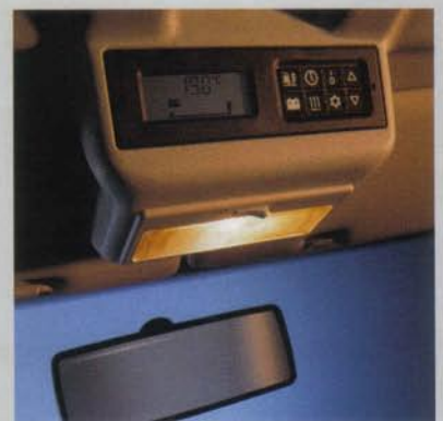
Im Blickfeld angeordnete Zentralelektronik mit Bedienung für Standheizung und Kühlbox.
