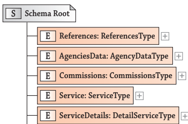
Elementos raíz del esquema XML STExtension v1.6.
