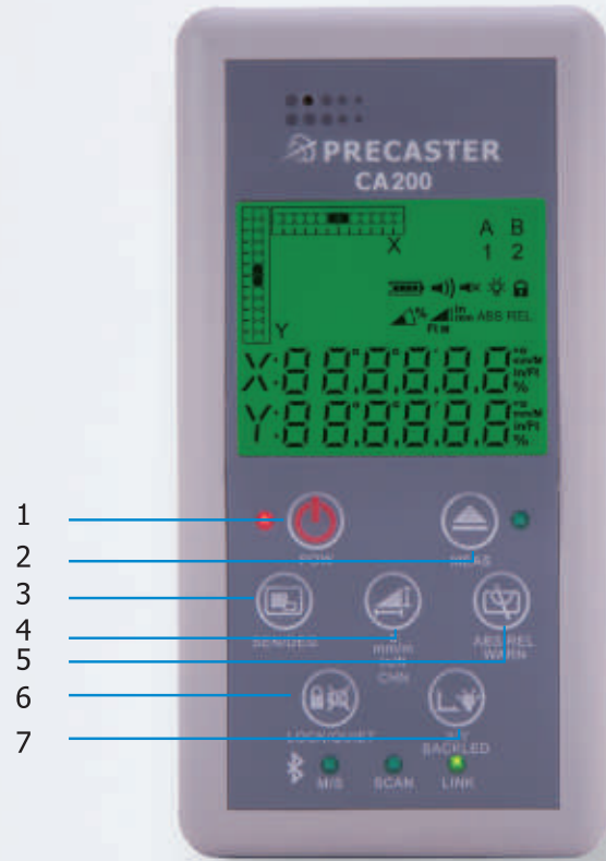
接收主機
