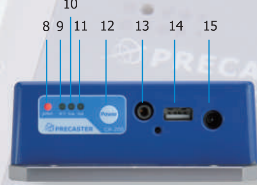
偵測副機
