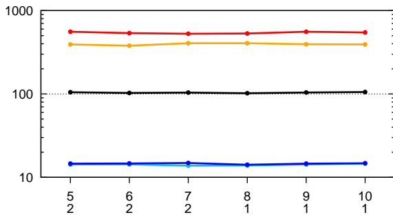
PAM30
