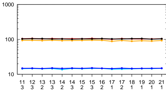
PAM250
