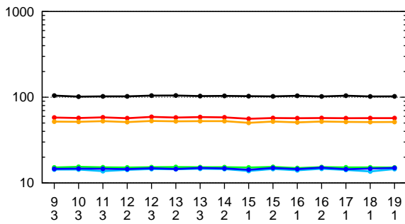
BLOSUM50
