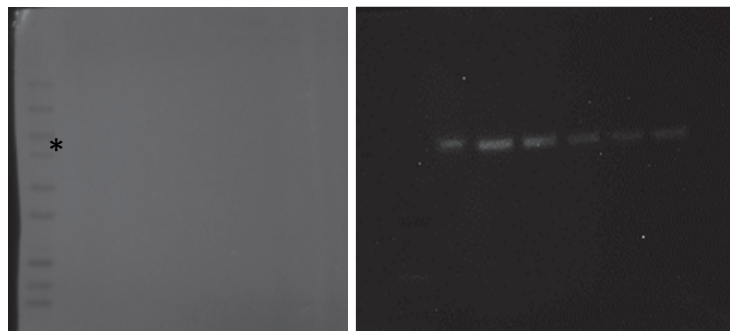
Fig. 3B STAT1
