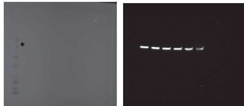
Fig. 3B STAT3
