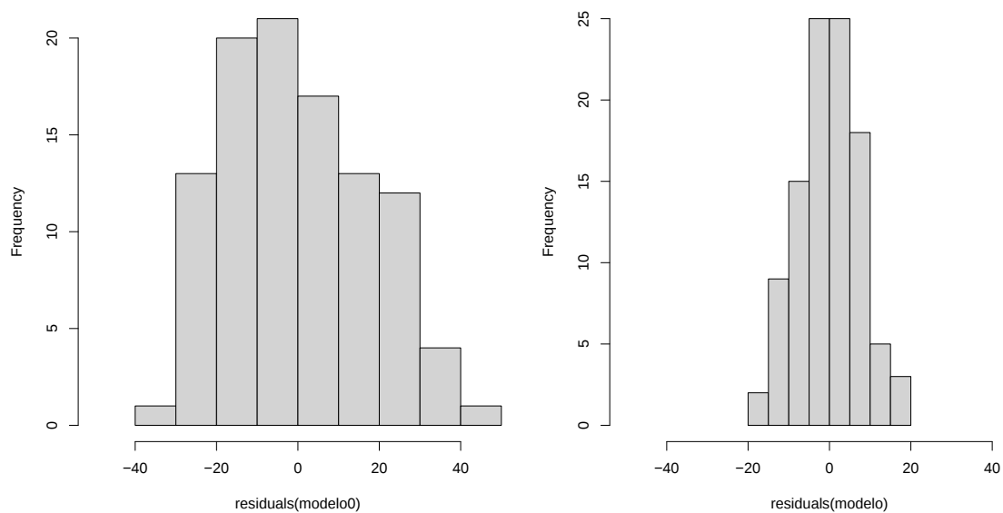
Figura 11.6: Variabilidad residual con el modelo reducido (izquierda) y con el modelo completo (derecha).
