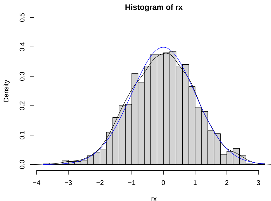
Figura 7.7: Distribución de los valores generados mediante remuestreo por importancia y densidad objetivo.
