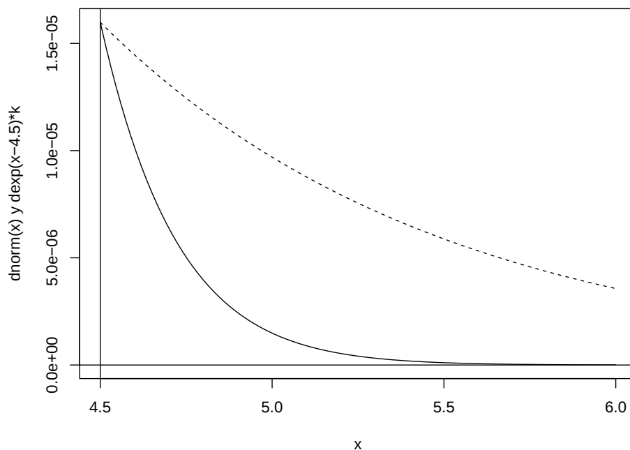
Figura 7.3: Objetivo a integrar (densidad objetivo truncada) y densidad auxiliar reescalada.
