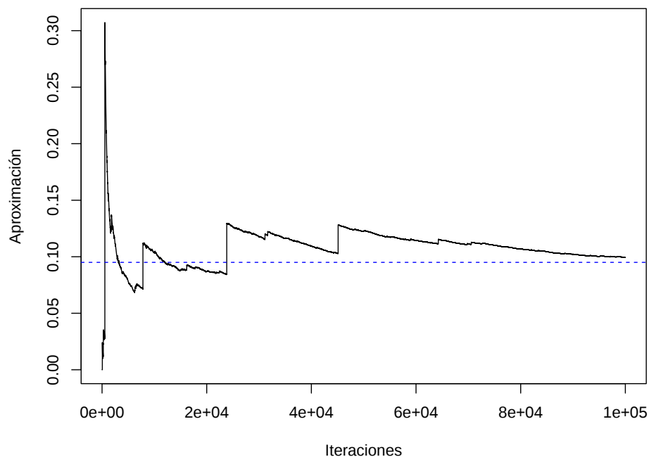
Figura 7.5: Gráfico de convergencia de la aproximación mediante muestreo por importancia con mala densidad auxiliar.
