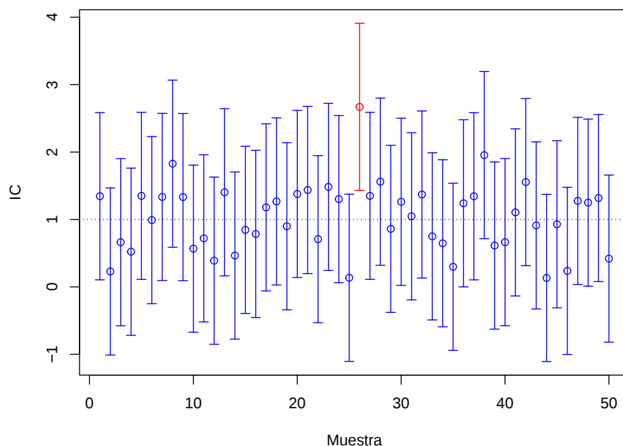
Figura 7.11: Cobertura de las estimaciones por IC.
