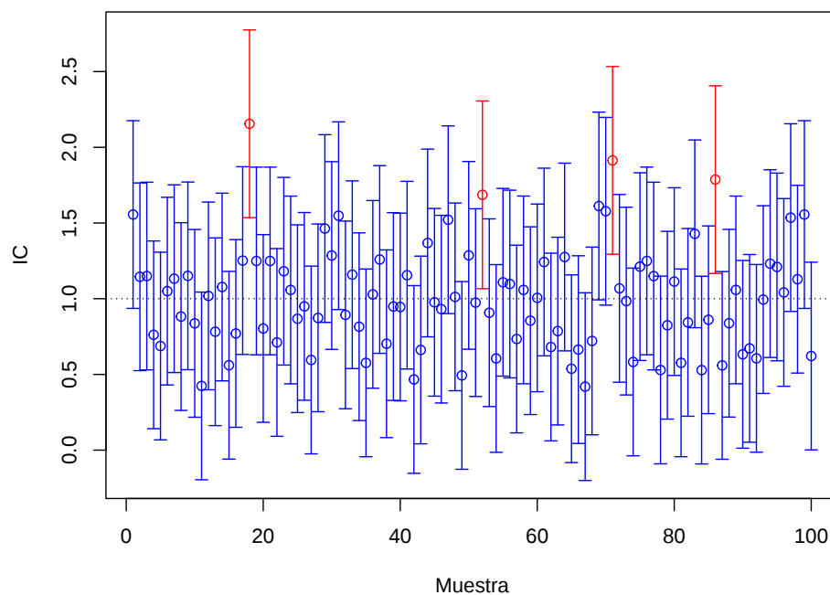
Figura 7.12: Cobertura de las estimaciones por IC (bajo normalidad).
