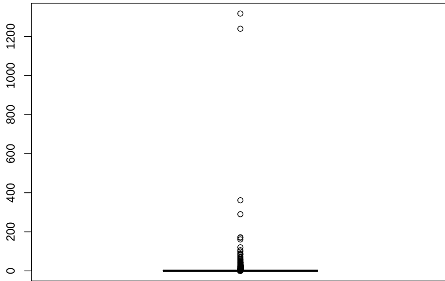
Figura 7.6: Gráfico de cajas de los pesos del muestreo por importancia reescalados (de forma que su media es 1).
