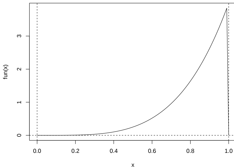
Figura 7.1: Ejemplo de integral en dominio acotado.
