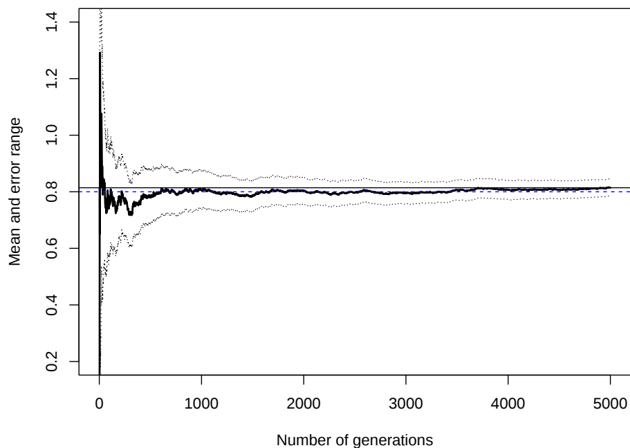
Figura 7.2: Convergencia de la aproximación de la integral mediante simulación.
