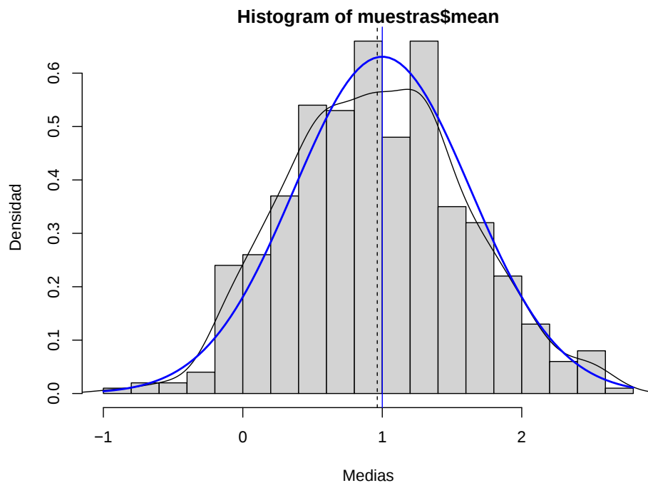
Figura 7.9: Distribución de la media muestral de una distribución normal.
