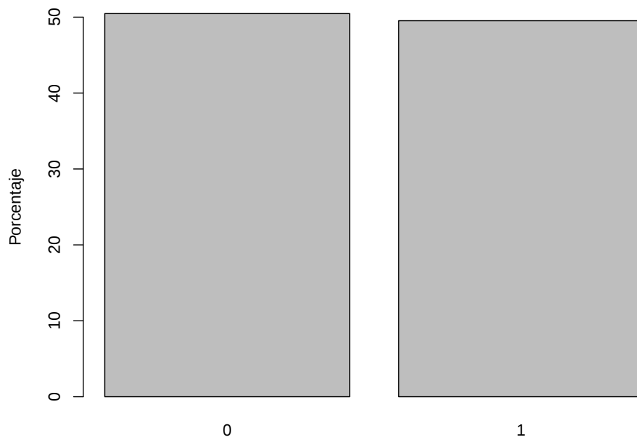
Figura D.2: Frecuencias relativas de los valores generados con distribución Bernoulli (aproximaciones por simulación de las probabilidades teóricas).
