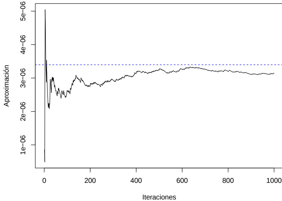
Figura 7.4: Convergencia de la aproximación de la integral mediante muestreo por importancia.
