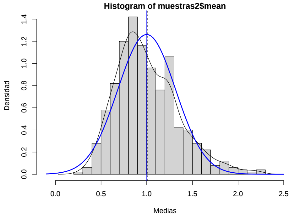
Figura 7.10: Distribución de la media muestral de una distribución exponencial y distribución asintótica.
